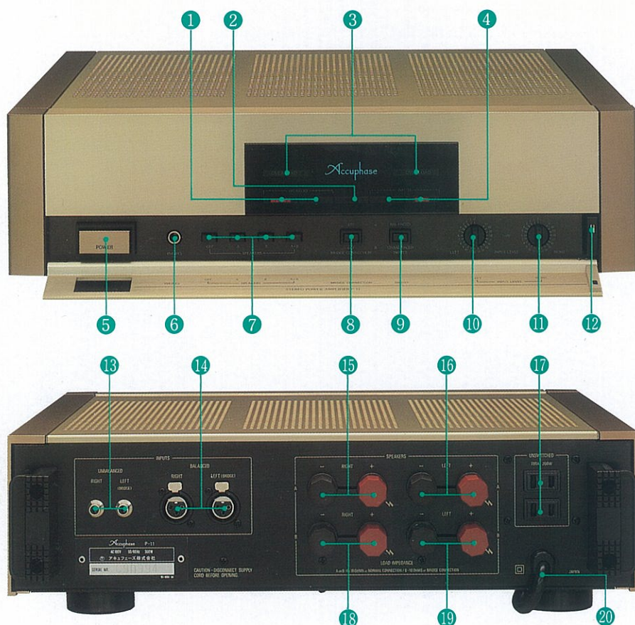
■ P-11 フロント・リアパネル
