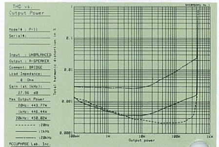
●P-II 全高調波ひずみ率/出力特性(8Ω負荷、モノフォニック仕様時)
