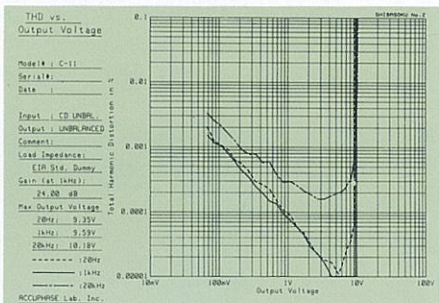
●C-II 入力電圧/全高調波ひずみ率(入力:CD不平衡/出力:不平衡端子)
