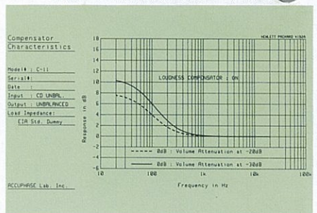
●C-II コンペンサター特性
