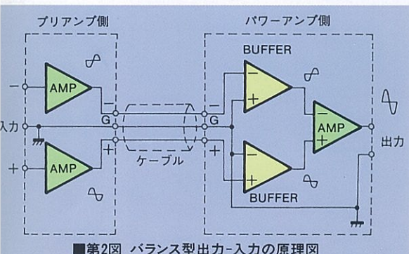
■第2図 バランス型出力-入力の原理図
