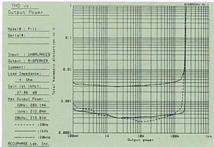
●P-II 全高調波ひずみ率/出力特性(4Ω負荷、ステレオ仕様時)
