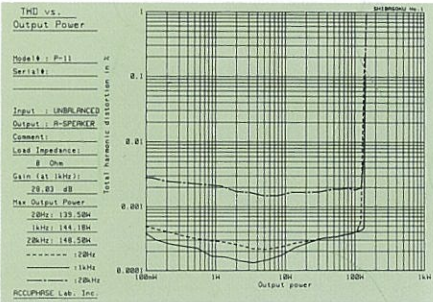
●P-II 全高調波ひずみ率/出力特性(8Ω負荷、ステレオ仕様時)
