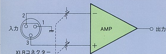
■第3図 P-11のバランス入力回路
