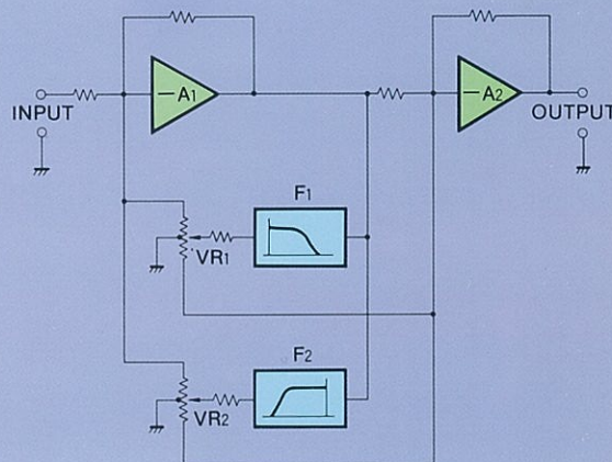
■第5図 トーン・コントロール回路の原理図 (加算型アクティブ・フィルター方式)
